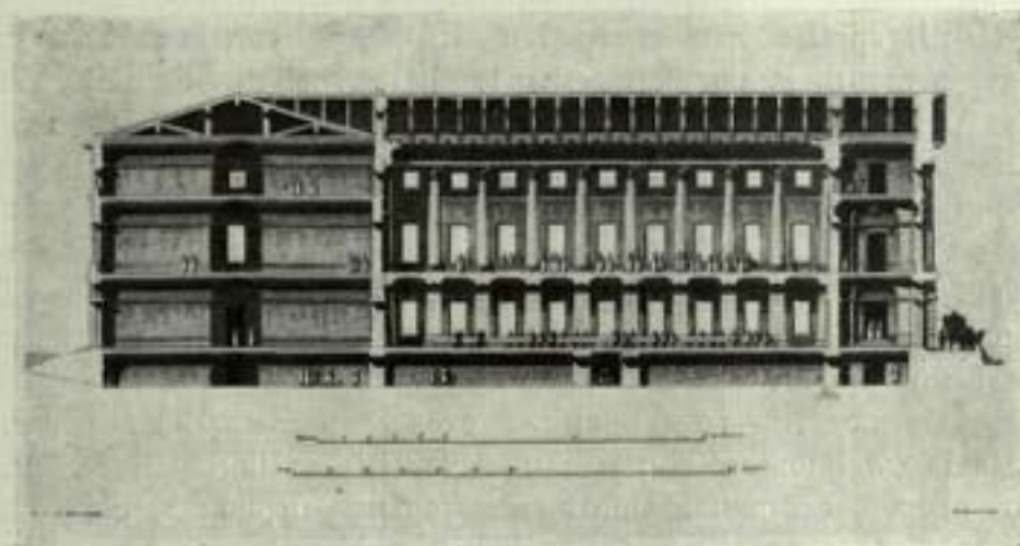
Разрѣзь новаго зданія.
