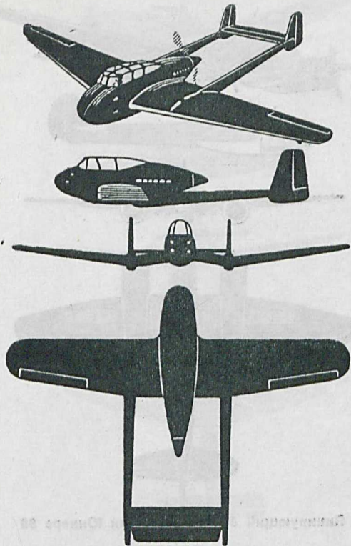
Истребитель Фокке-Вульф 198
