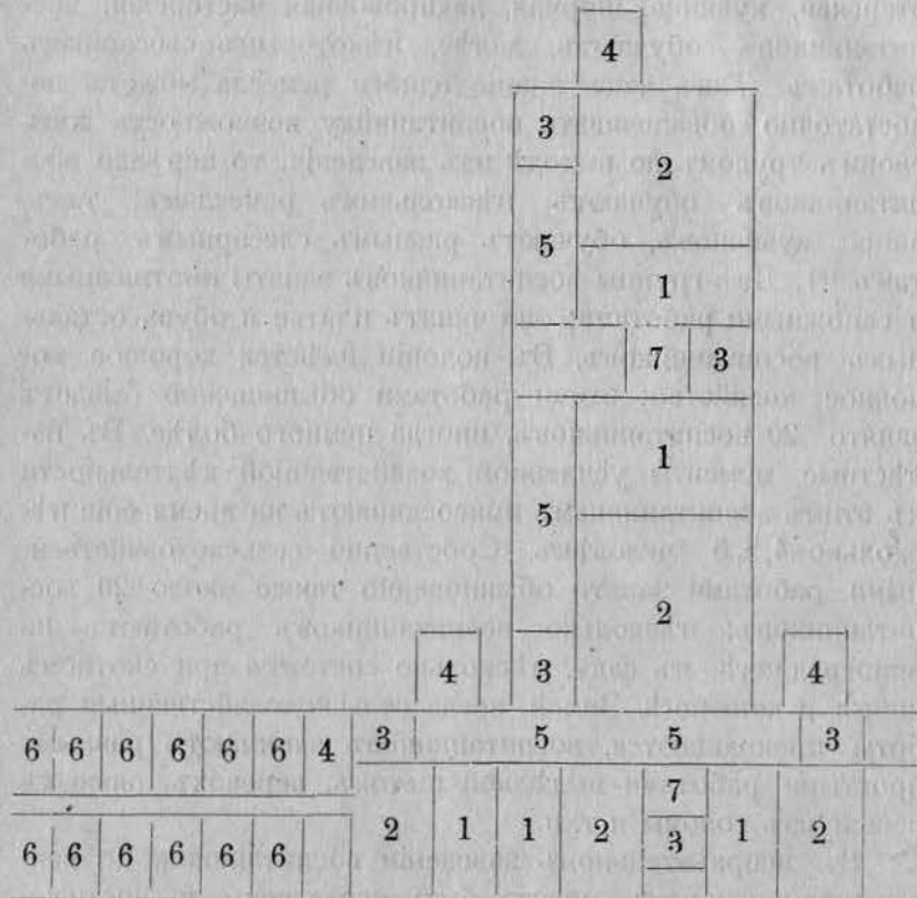
Планъ верхняго этажа.
