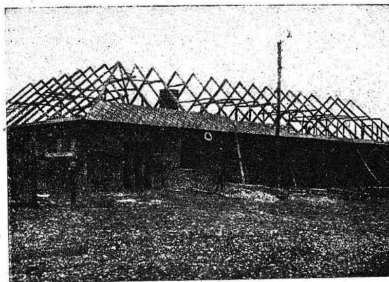
Рис. 8. С.-х. коммуна «Искра» строит электростанцию (Шевченковский окр.)
