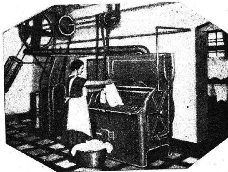
Рис. 22. Механическая прачечная
