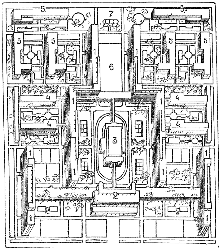
Из материалов Сталинградстроя. Проект жилого комбината архитекторов А. и Л. ВЕСНИНЫХ.
