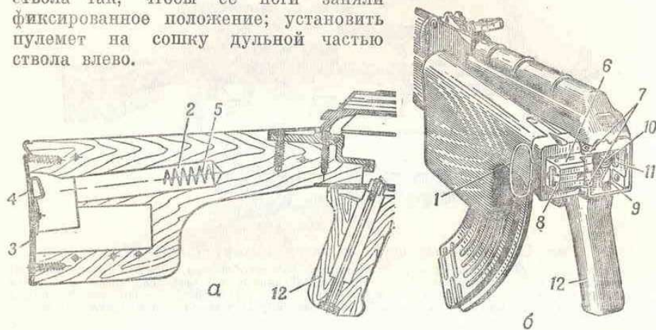
Рис. 126. Приклад и pistolетная рукоятка:
