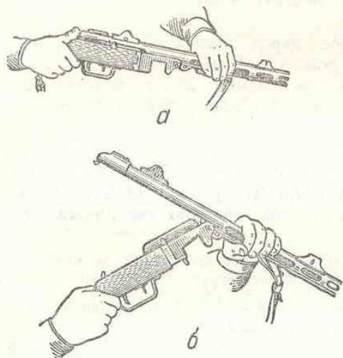
Рис. 80. Открывание затворной коробки: а — утапливание колпачка; б — опускание кожуха
