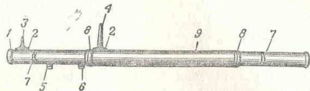
Рис. 129. Ствол:
