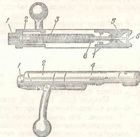
Рис. 150. Затвор:
