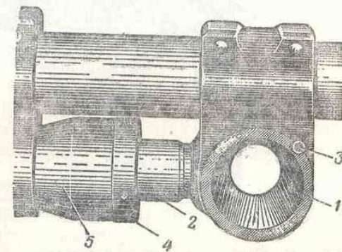
Рис. 108. Газовая камера:
