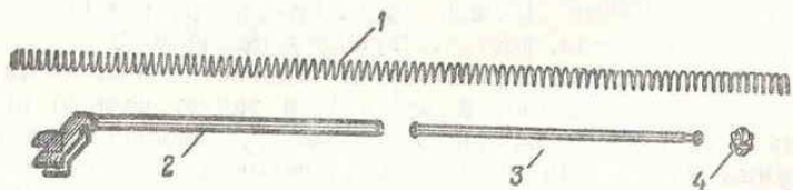
Рис. 71. Возвратный механизм:
