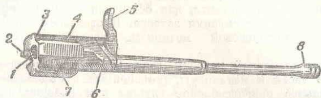
Рис. 69. Затворная рама с газовым поршнем:
