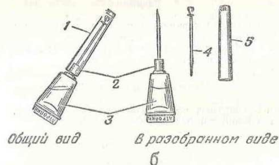
Рис. 45, а, б. Шприц-тюбики двух типов: 1 — колпачок; 2 — горловина; 3 — корпус; 4 — игла; 5 — колпачок; 6 — мембрана
