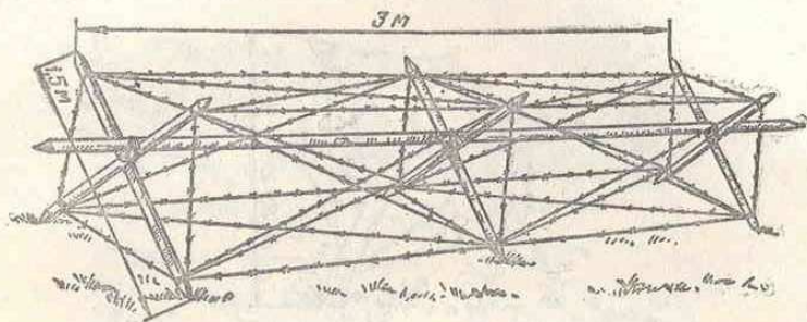
Рис. 32. Рогатка
