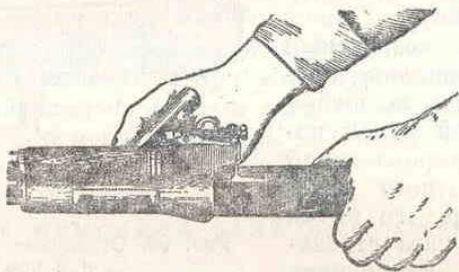
Рис. 64. Поворот замыкателя газовой трубки с помощью пенала принадлежности
