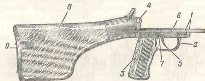
Рис. 120. Спусковая рама с прикладом:
