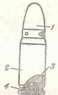
Рис. 87. Боевой патрон: 1 — пуля; 2 — гильза; 3 — заряд; 4 — капсюль
