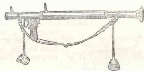
Рис. 127. Общий вид ручного противотанкового гранатомета РПГ-2.
