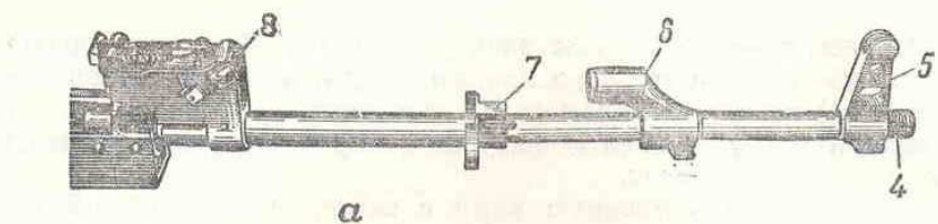
Рис. 66. Ствол:
