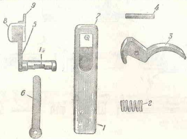
Рис. 121. Спусковой механизм:
