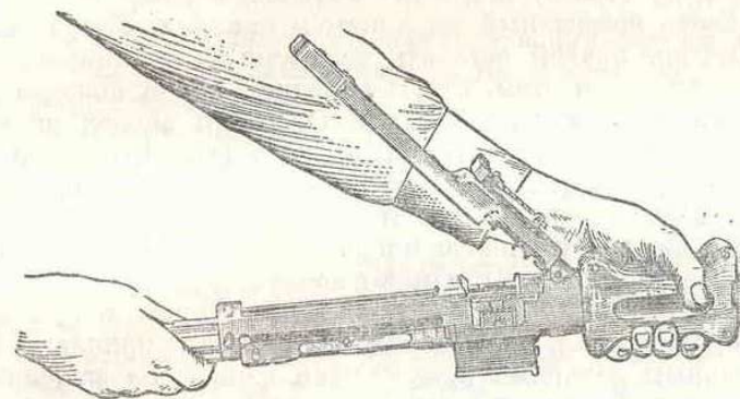
Рис. 106. Отделение затворной рамы
