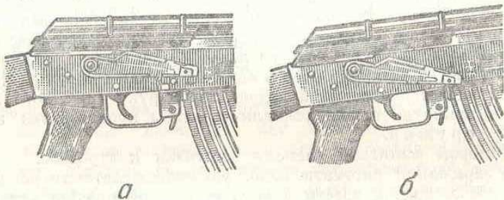
Рис. 90. Постановка переводчика на необходимый вид огня: а — на автоматический огонь; б — на одиночный огонь
