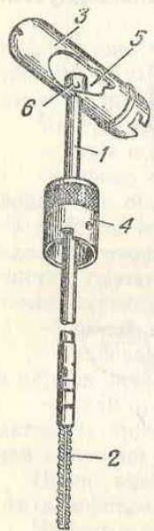
Рис. 158. Принадлежность автомата, подготовленная для чистки: 1 — шомпол; 2 — протирка; 3 — пенал; 4 — крышка пенала; 5 — отвертка; 6 — головка шомпола
