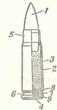
Рис. 76. Боевой патрон: 1 — пуля; 2 — гильза; 3 — пороховой заряд; 4 — капсюль; 5 — дульце; 6 — проточка; 7 — наковальня; 8 — затравочное отверстие; 9 — ударный состав
