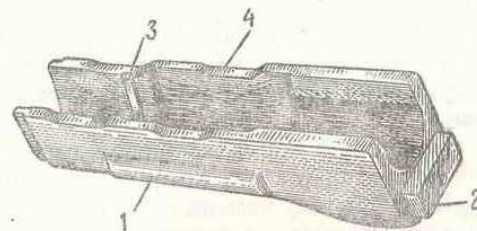
Рис. 73. Цевье:
