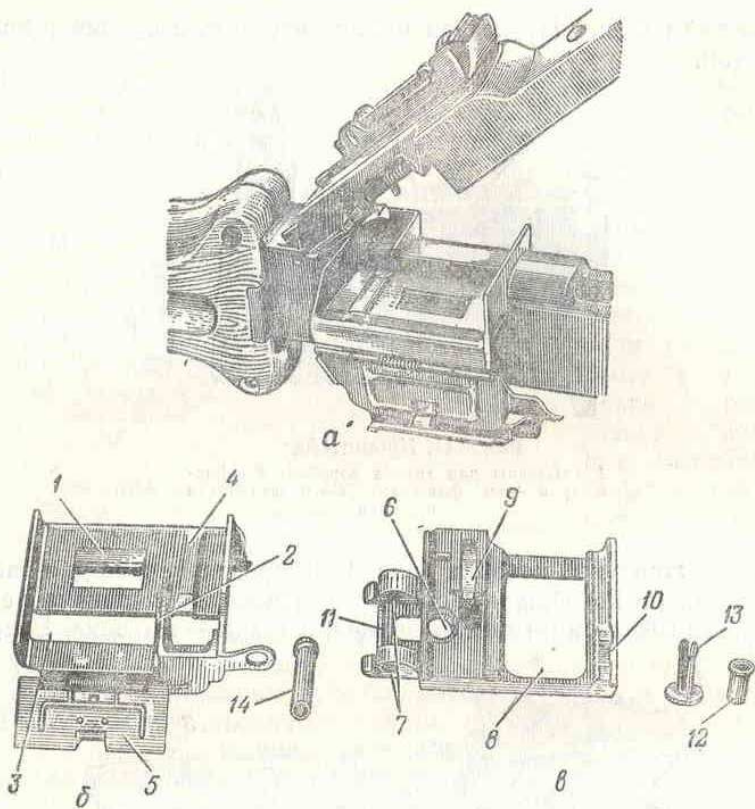
Рис. 113. Приемник:
