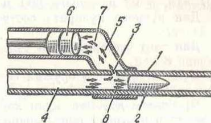
Рис. 46. Принцип работы автоматики:
