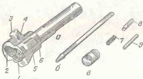
Рис. 70. Затвор:
