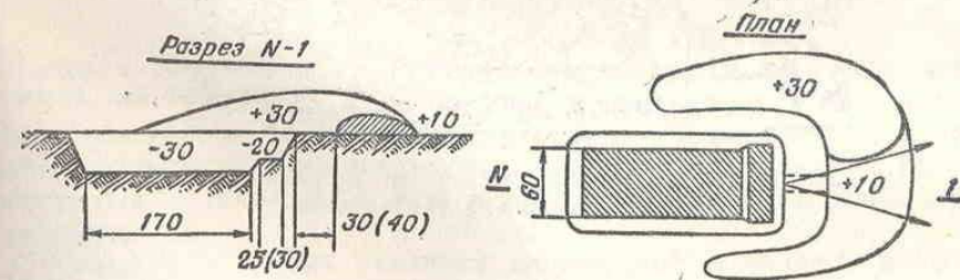
Рис. 35. Одиночный окоп для стрельбы из автомата лежа
