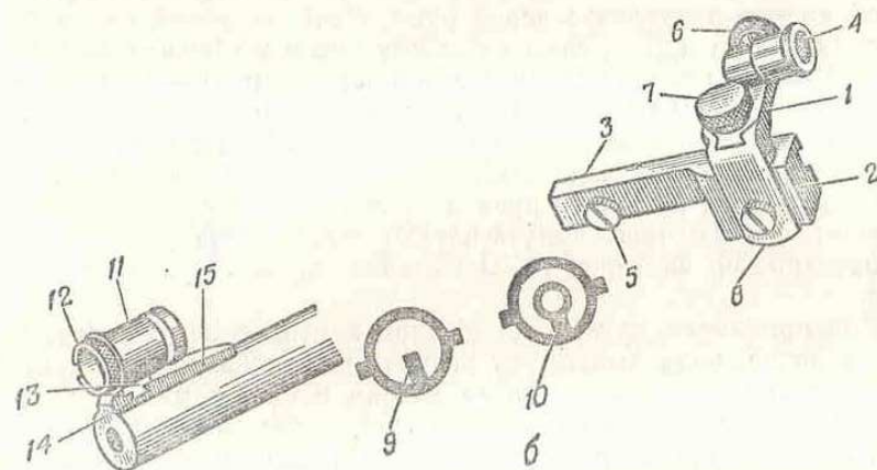
Рис. 154. Малокалиберная винтовка ТОЗ-12:
