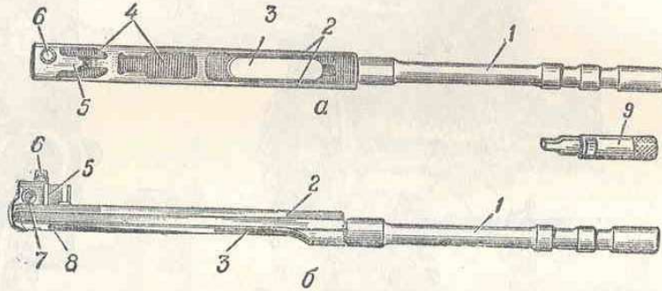
Рис. 117. Затворная рама с газовым поршнем:
