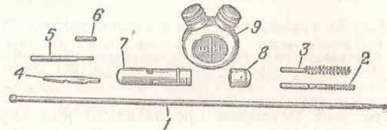
Рис. 75. Принадлежность: 1 — шомпол; 2 — протирка; 3 — ершик; 4 — отвертка; 5 — выколота; 6 — щипелька; 7 — пенал; 8 — крышка; 9 — масленка
