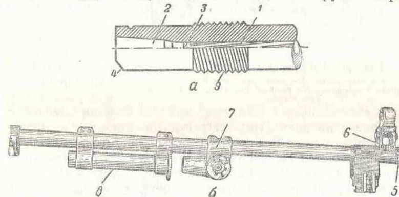
Рис. 107. Ствол:
