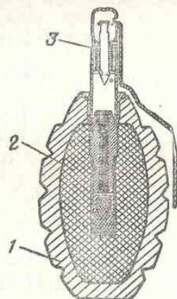
Рис. 164. Устройство ручной осколочной гранаты Ф-1:
